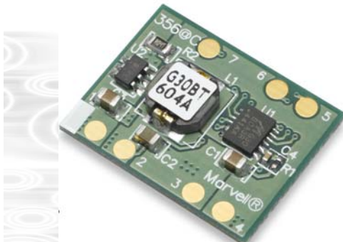
SMT Package
